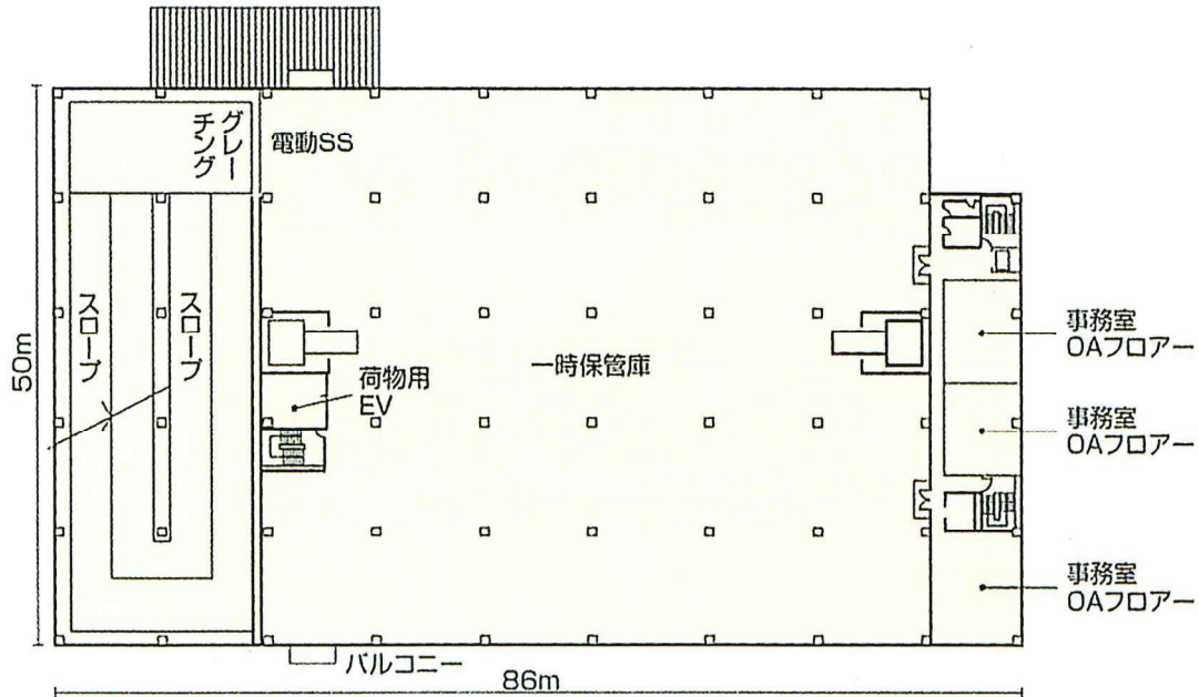
2F~5F 平面図
