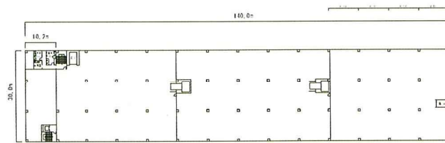
5F 平面図
