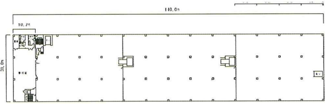
4F 平面図
