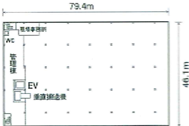
2F 平面図
