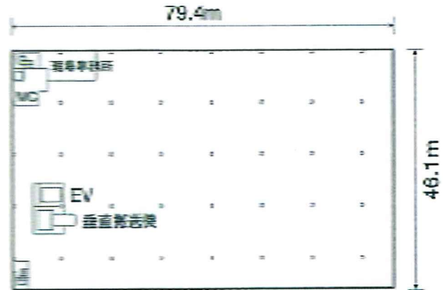
3F 平面図
