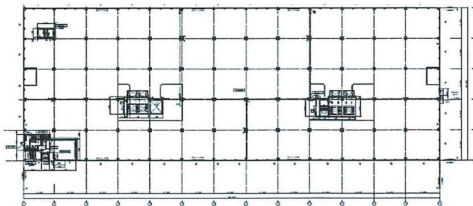
3F~5F 平面図
