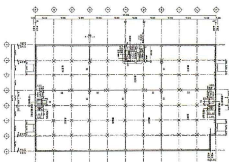
3F 平面図
