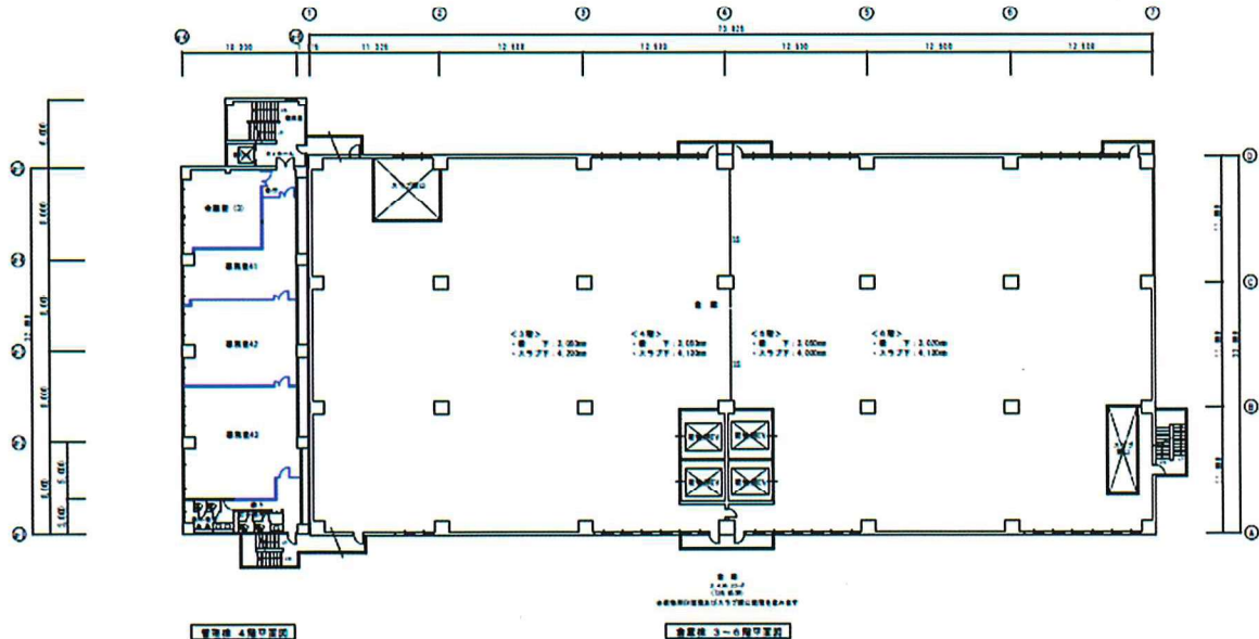
3F~6F 平面図
